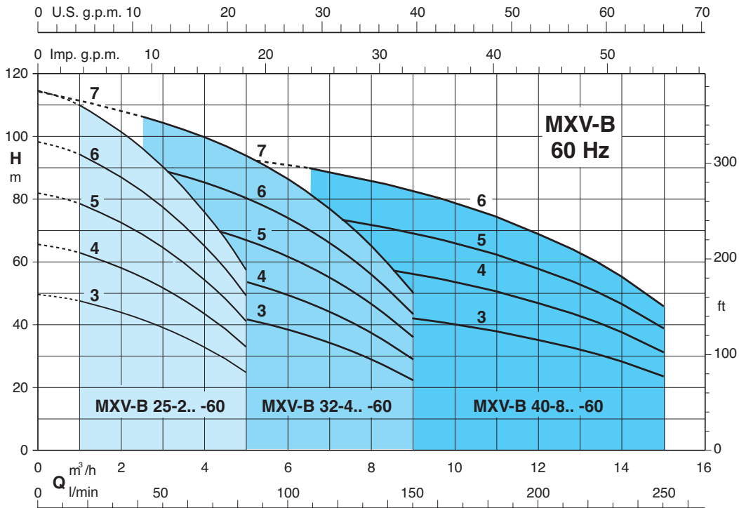
Coverage chart - Campo de aplicaciones n ≈ 3450 rpm
